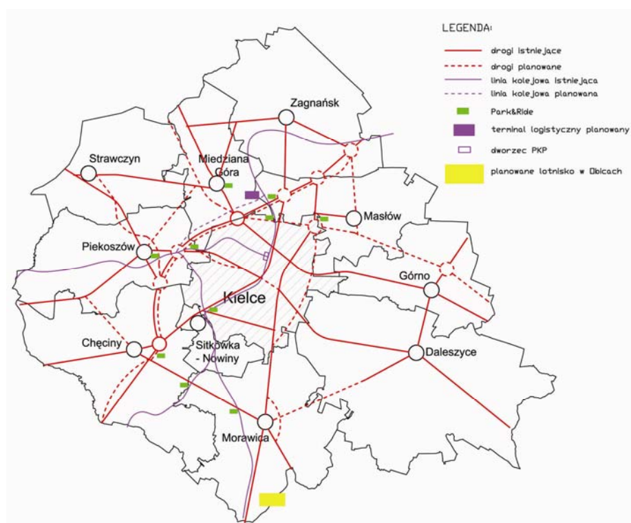
Rys. 13-1. Model struktury systemu transportowego Kieleckiego Zespołu Metropolitalnego – opcja z koleją regionalną
